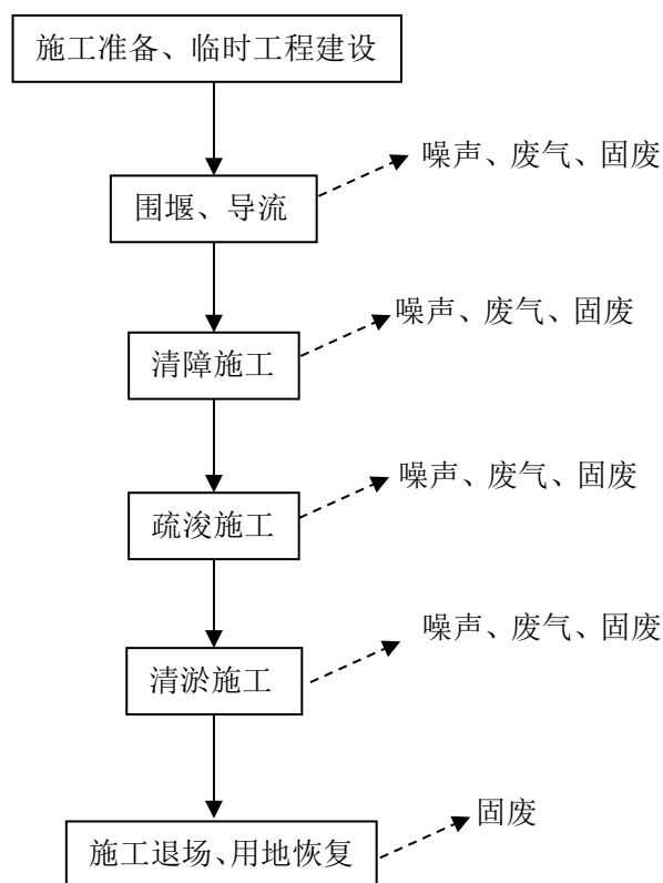
图 2-2 施工期工艺流程及产污环节图
