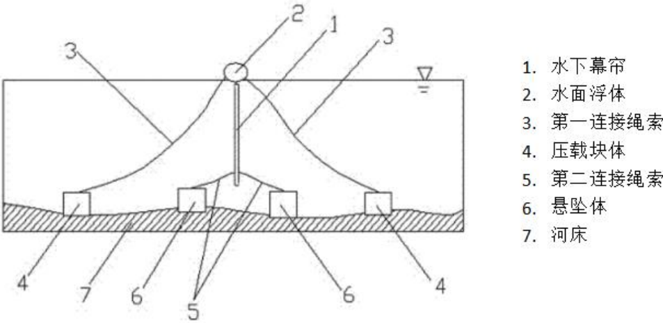
图 5-1 防泥幕帘制作图
