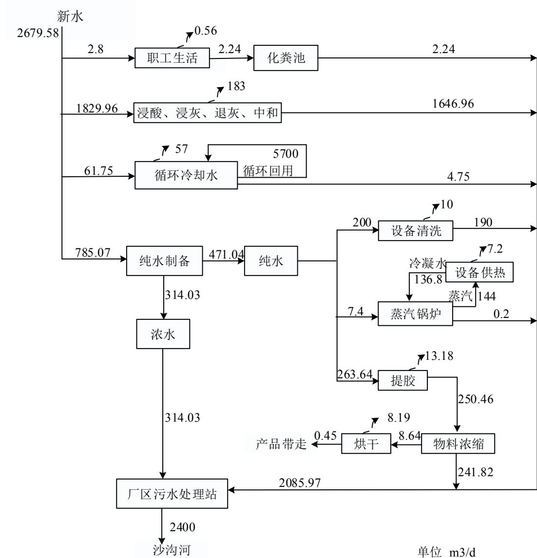
图 1-1 现有工程水平衡图
