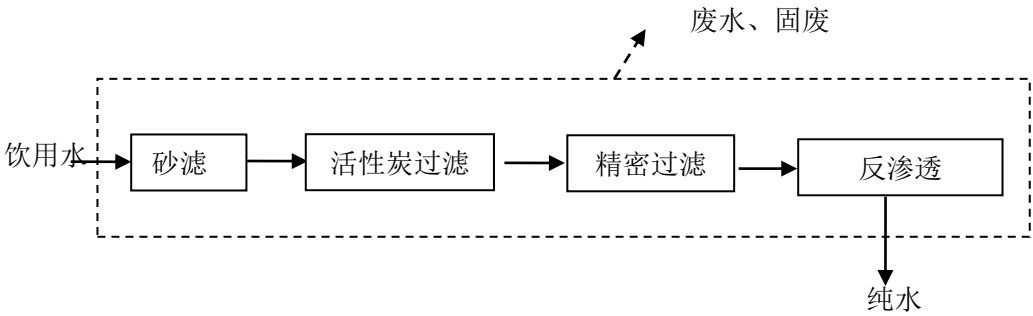
图 2-3 纯水制备工艺流程图及产污环节图
