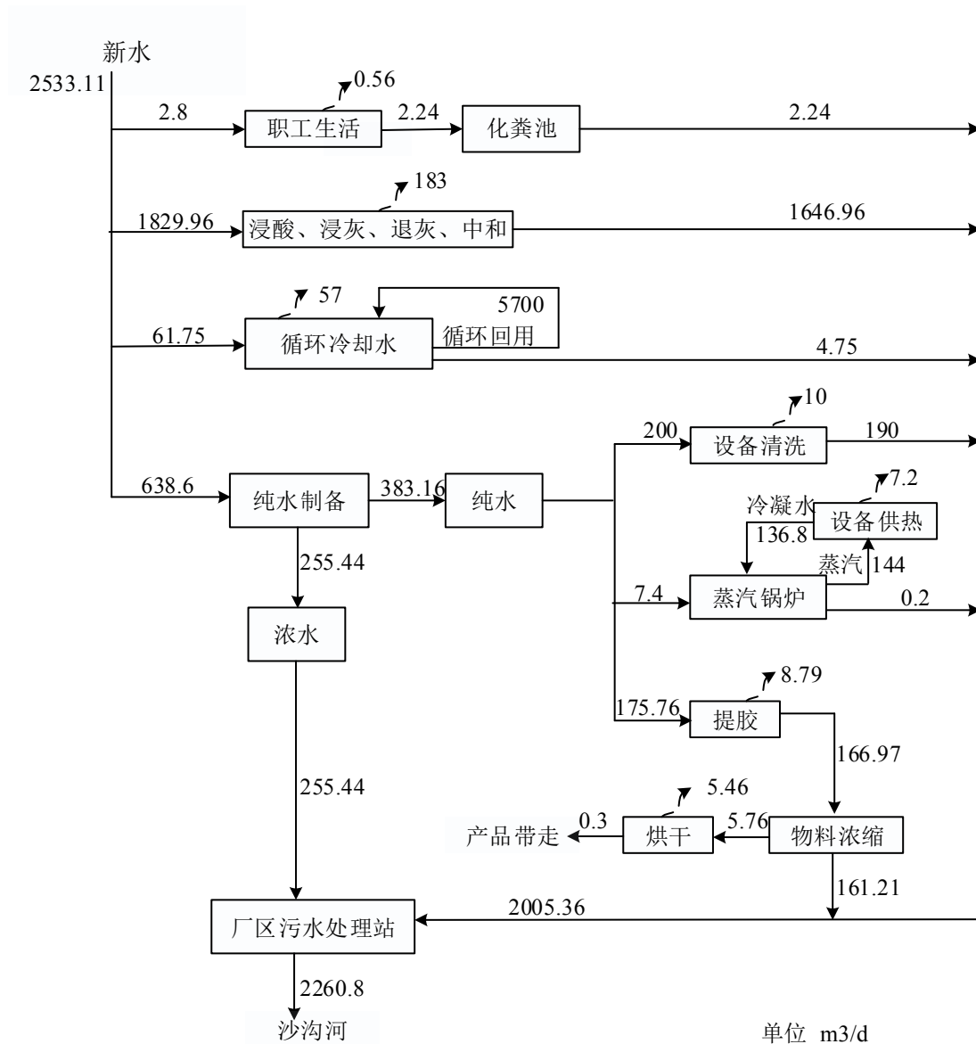
图 1-3 改建后现有工程水平衡图
