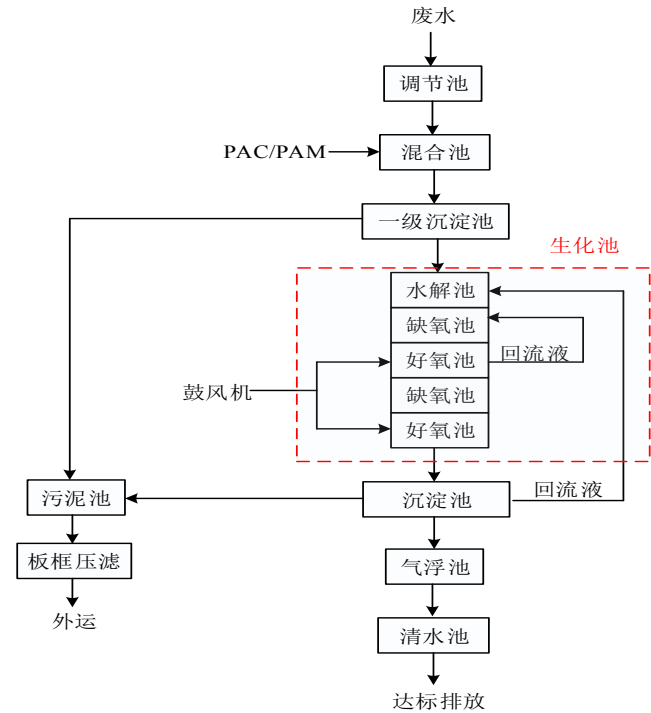
图 1-4 废水处理站工艺流程
