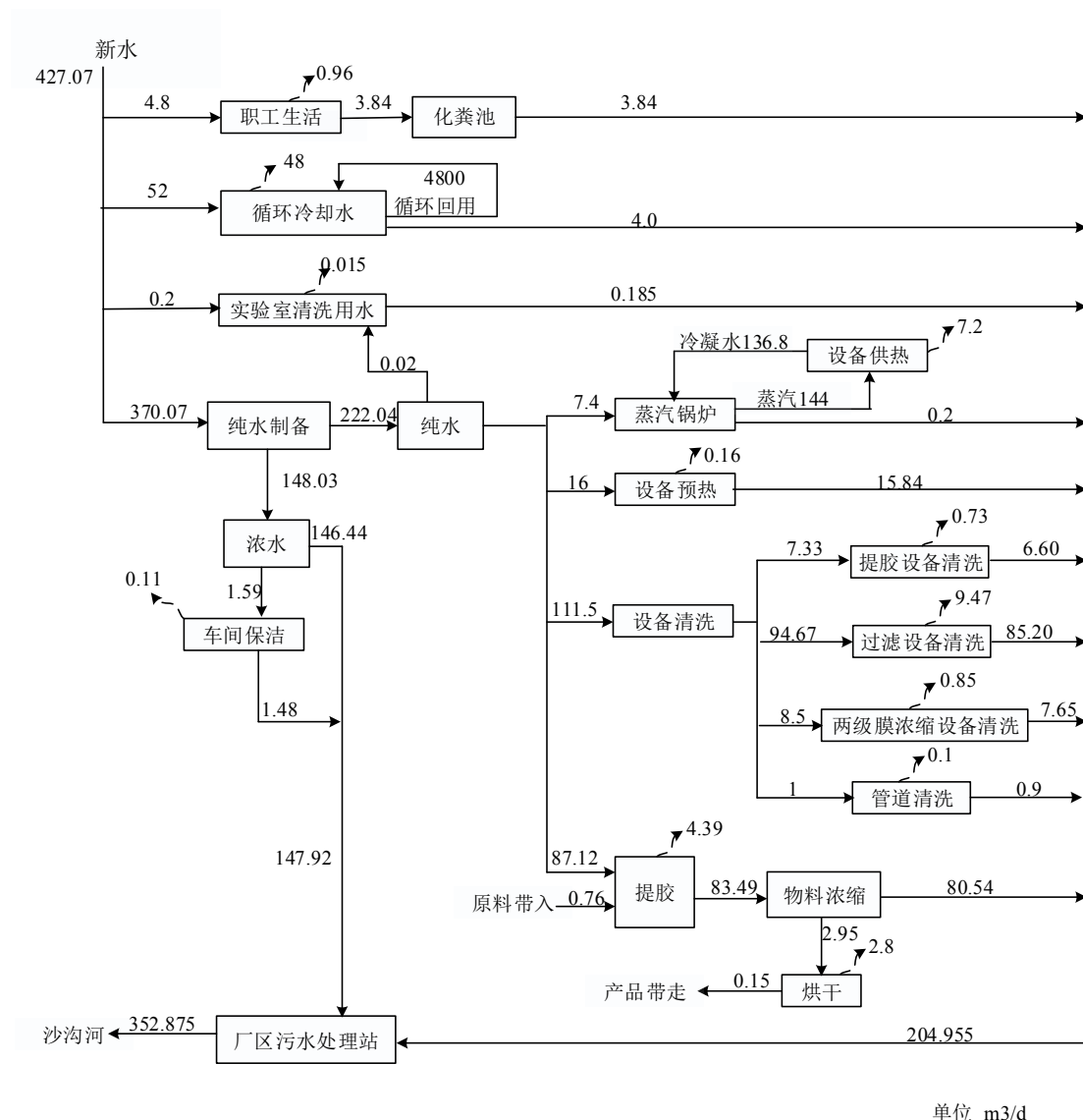
图 1-2 改建工程水平衡图
