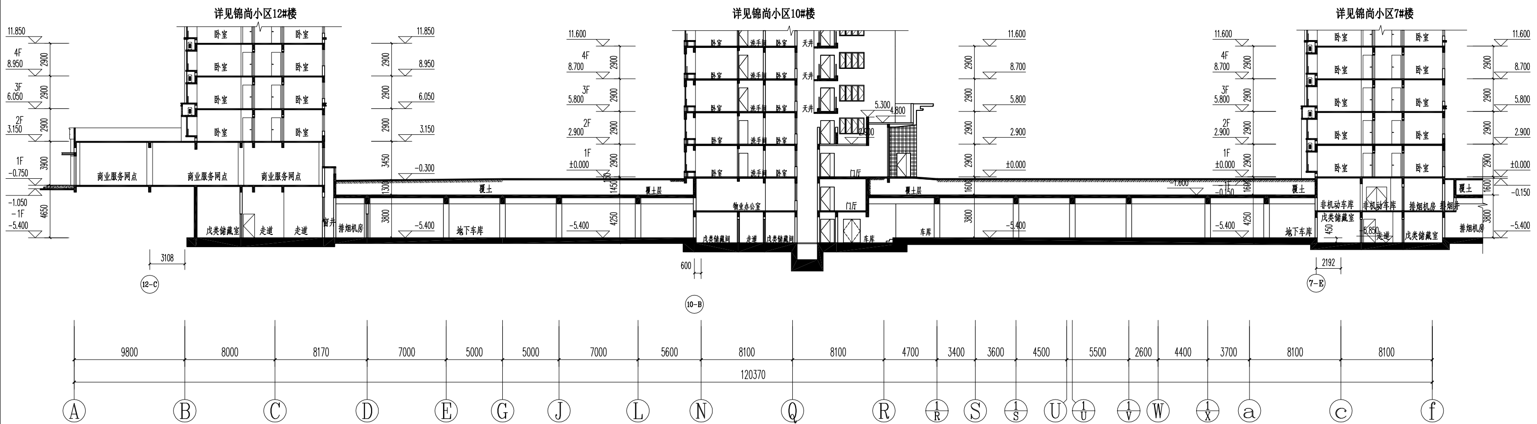
1-1 剖面图 (左半部分) 1:200
