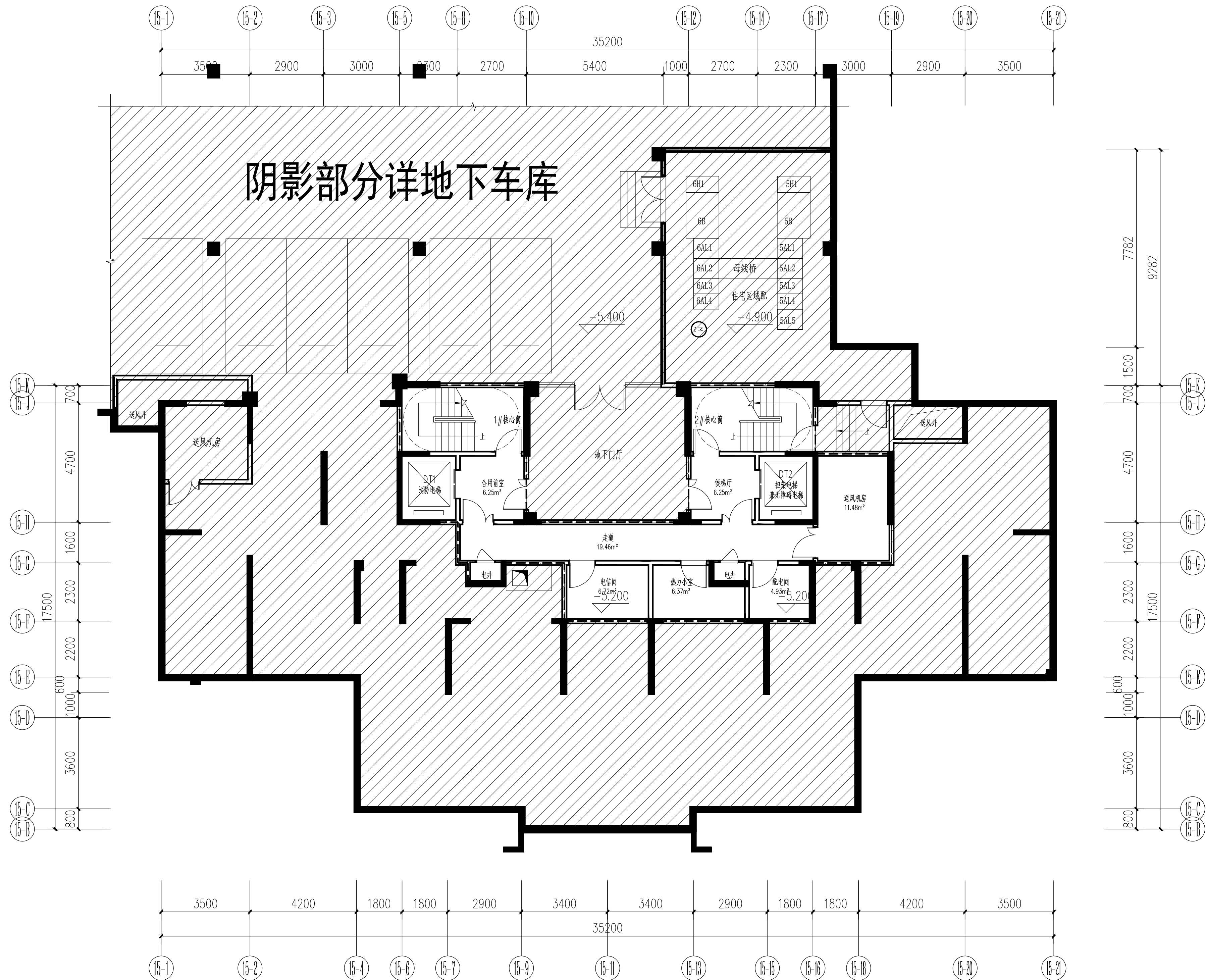
地下一层平面图 1:100 -5.400 本层建筑面积: 113.12m 2
