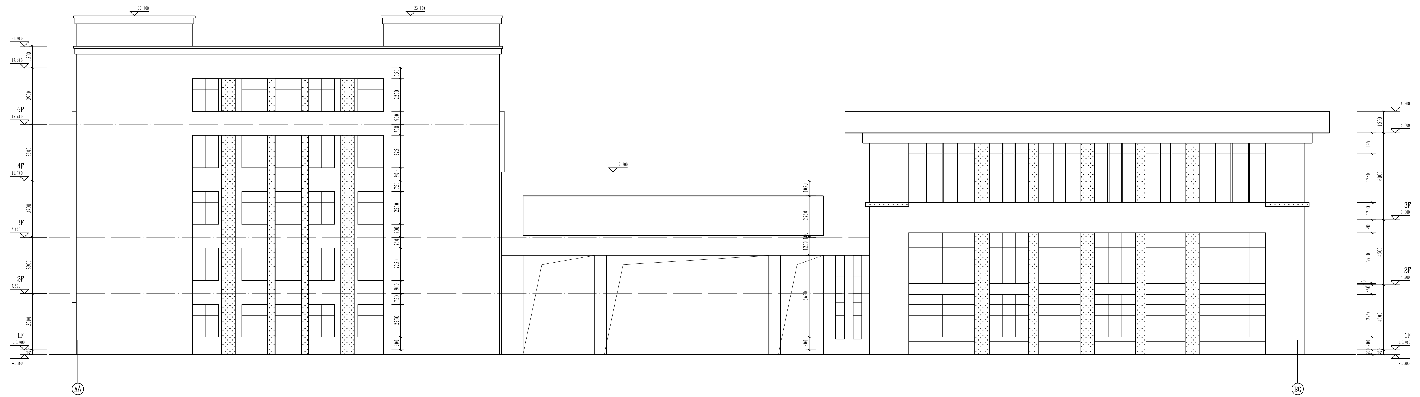
实训基地东立面图 1:150
