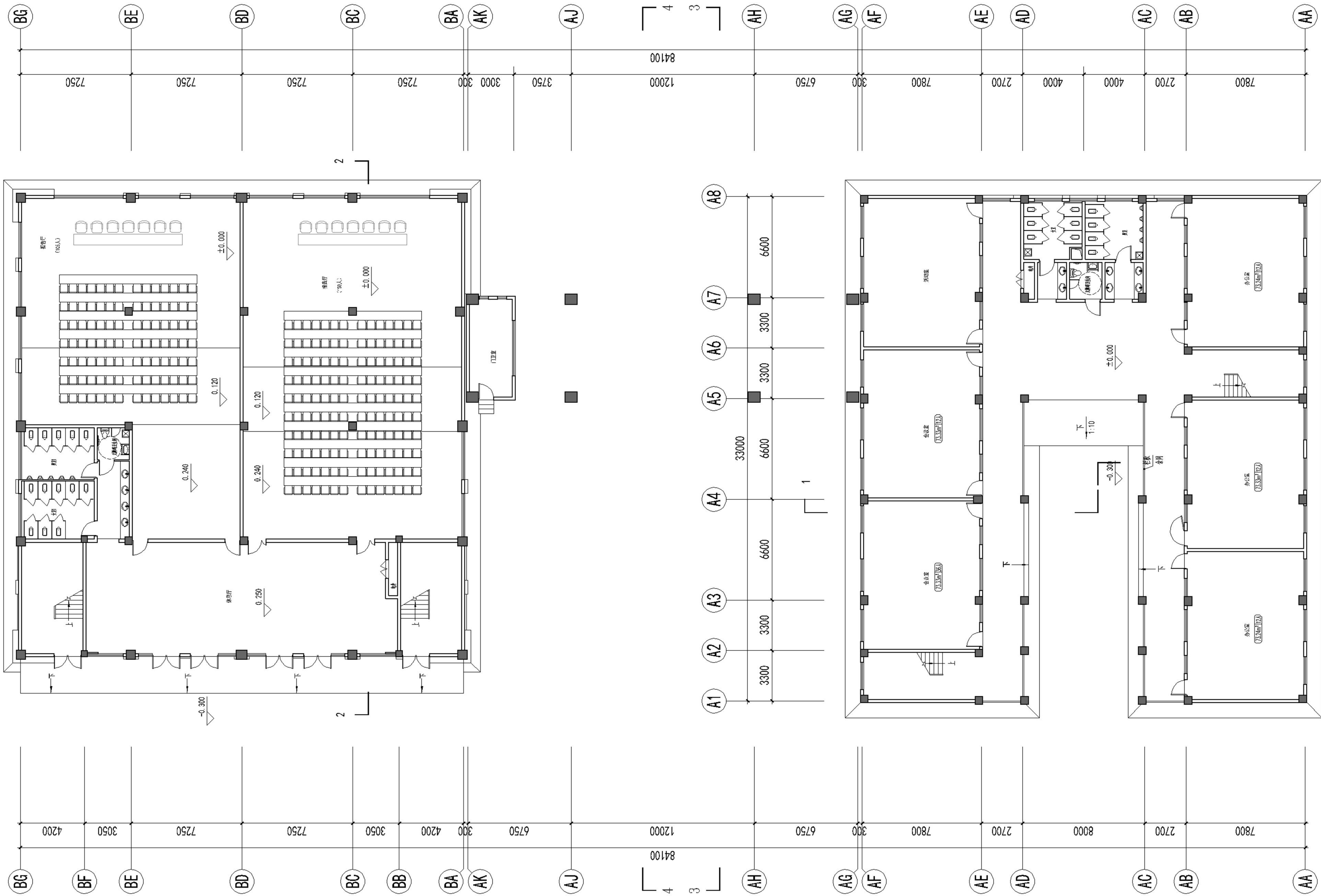
实训楼、报告厅一层组合平面图
