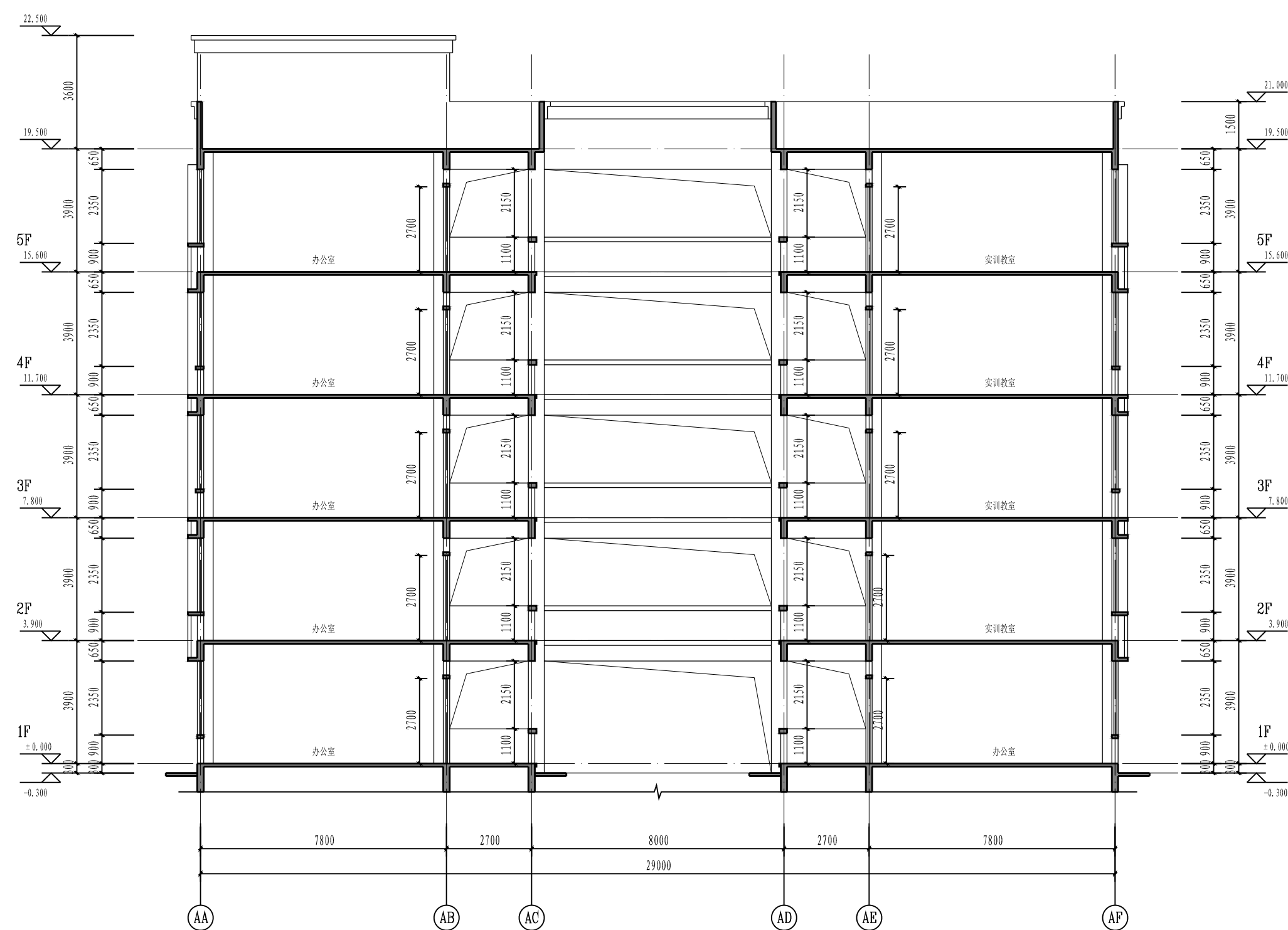
实训基地实训楼剖面图 1:150
