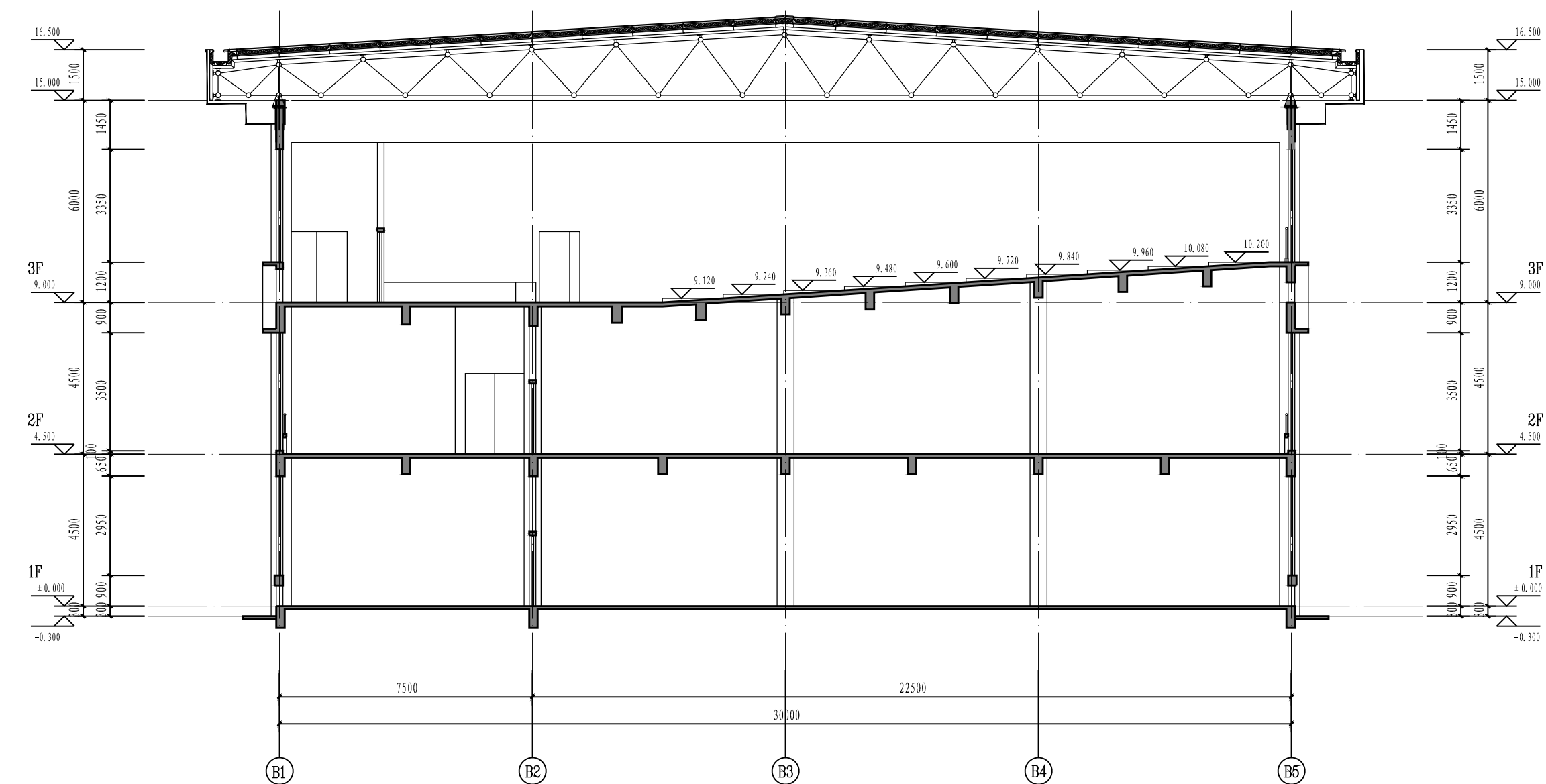
实训基地报告厅剖面图 1:150
