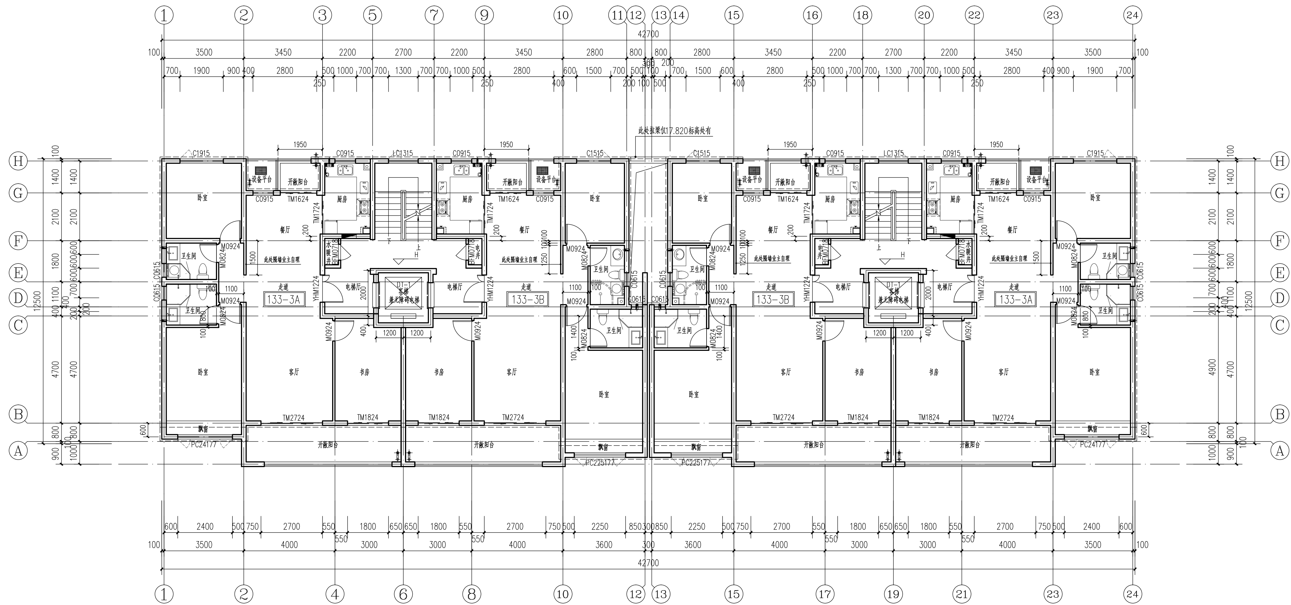
三~八层平面图 1:100
