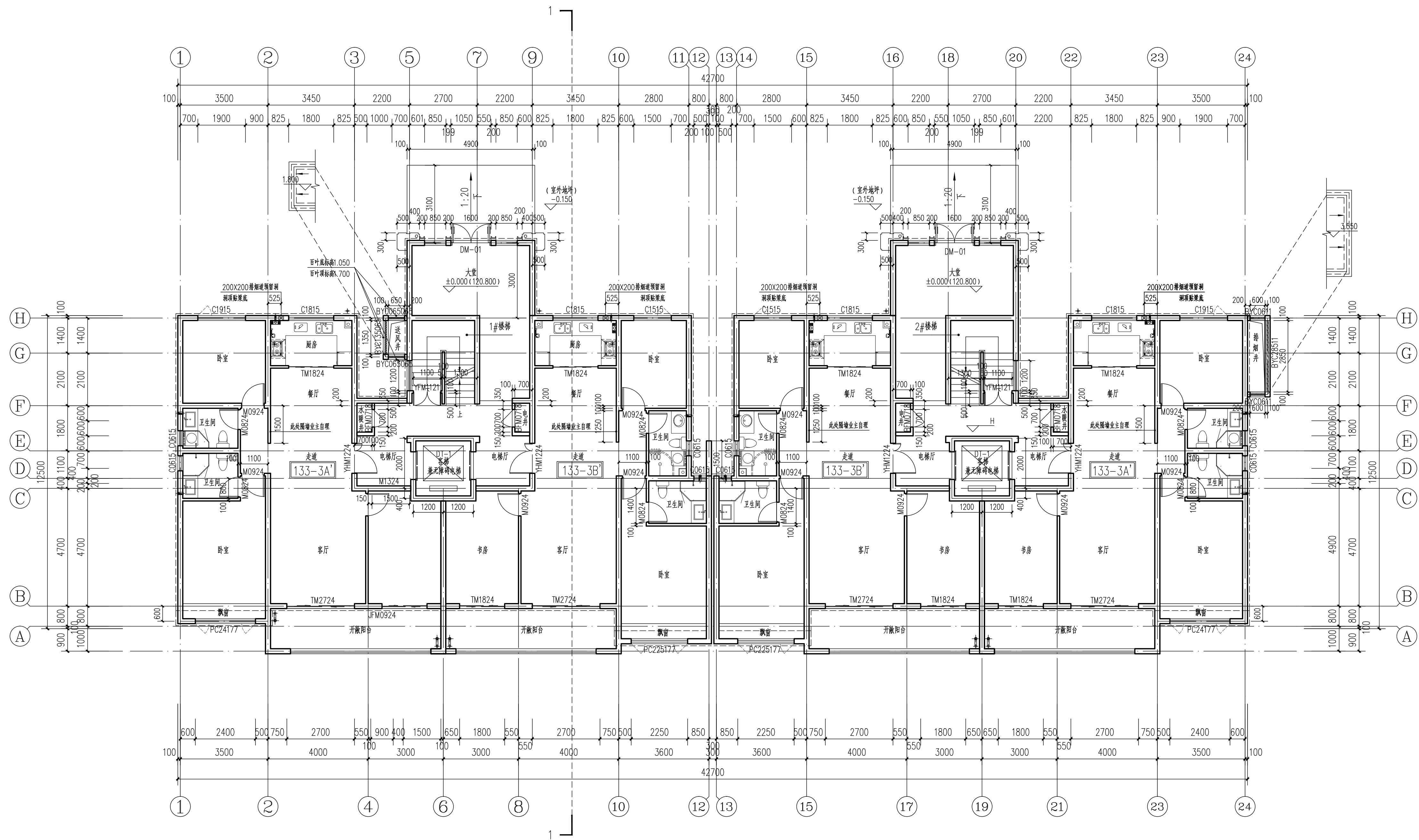
一层平面图 1:100
