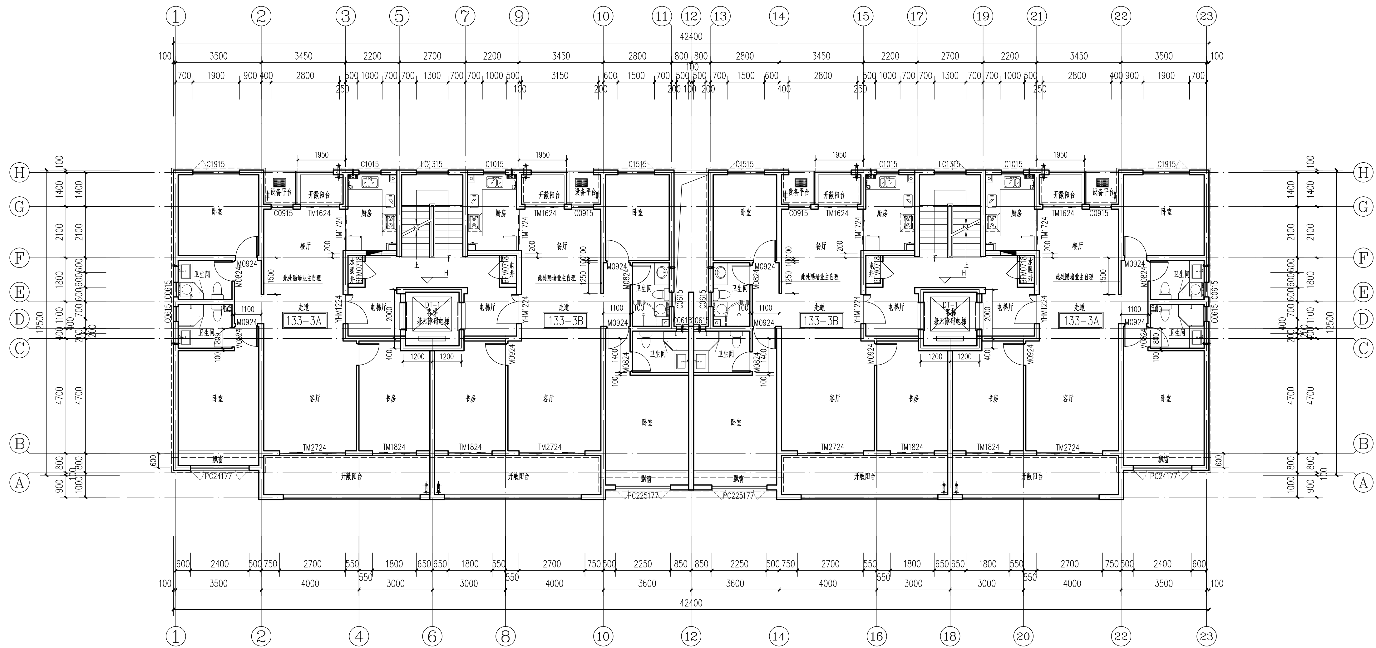
四~十一层平面图 1:100
