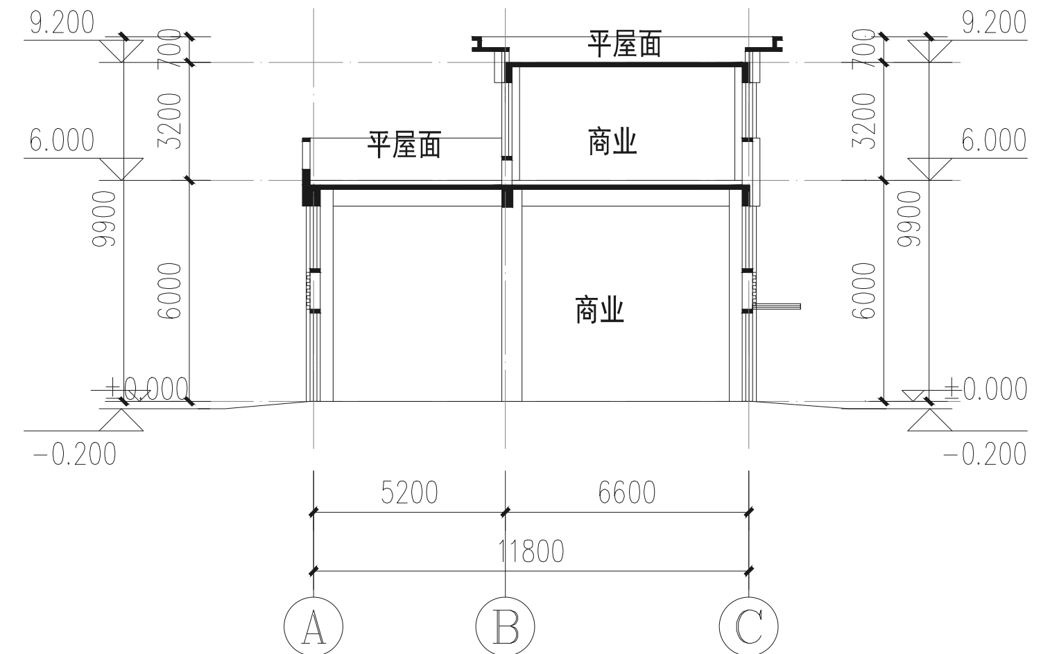
1-1剖面图 1:200
