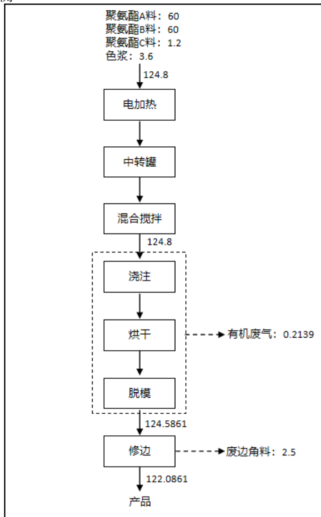
聚氨酯鞋底布鞋物料平衡图
