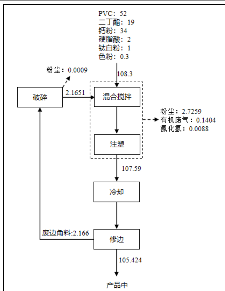
PVC 鞋底布鞋物料平衡图
