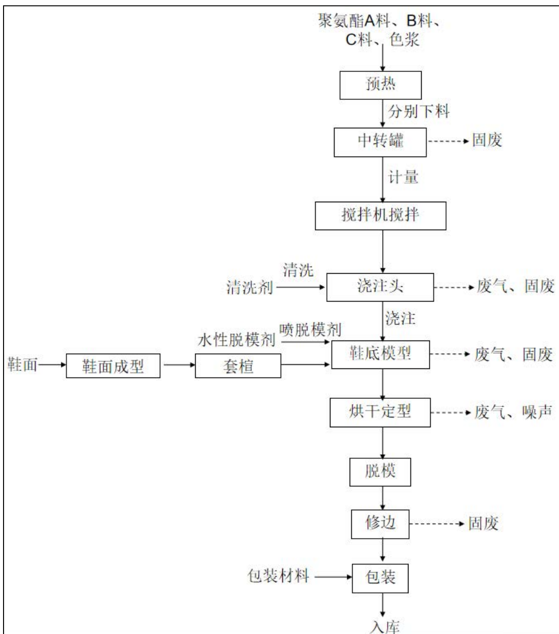
图 2-1 聚氨酯鞋底布鞋生产线工艺流程及产污环节图
