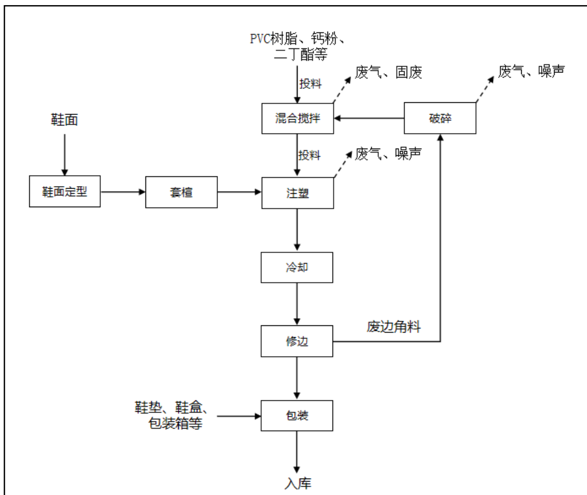
图 2-2 PVC 鞋底布鞋生产线工艺流程及产污环节图
