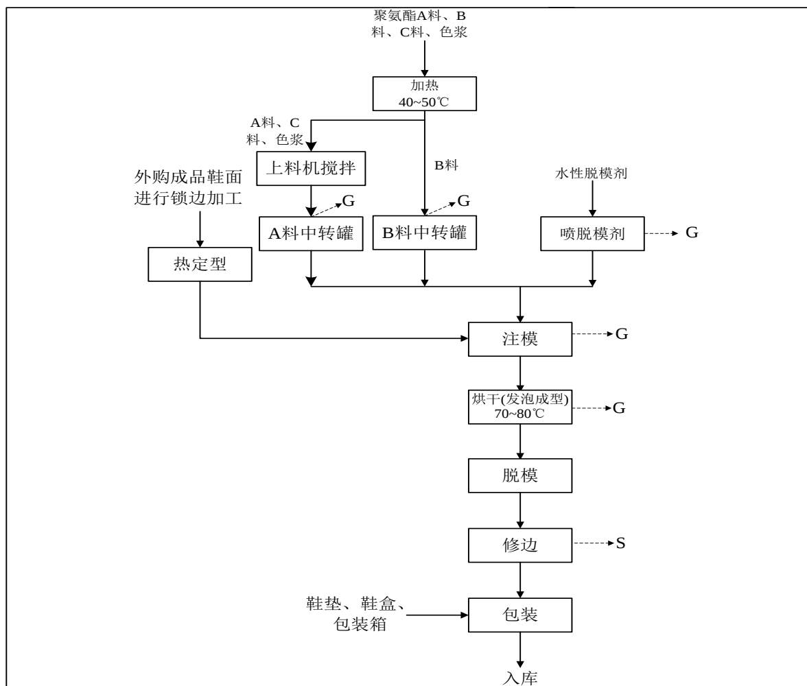
图 2-2 聚氨酯鞋底布鞋生产线工艺流程及产污环节图
