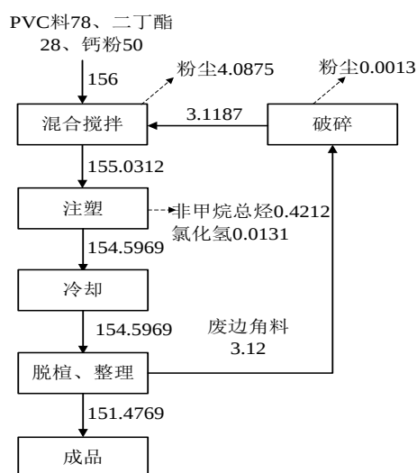
注塑工艺布鞋生产线-PVC 物料平衡图
