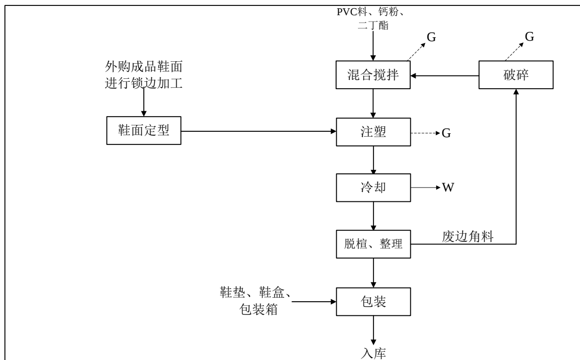
图 2-1 注塑工艺布鞋生产线工艺流程及产污环节图
