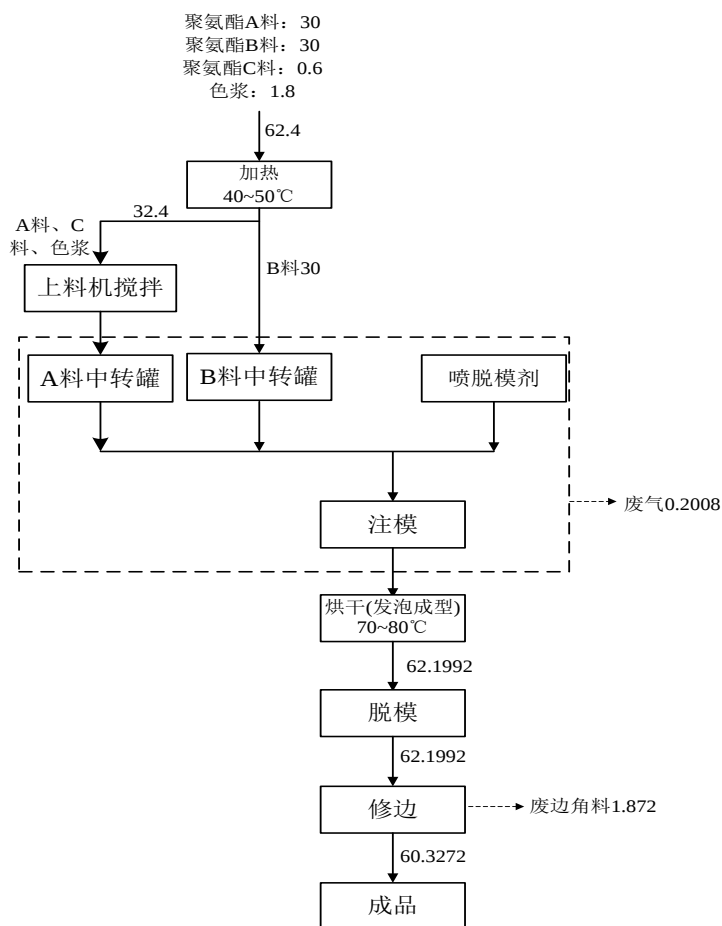
聚氨酯鞋底布鞋物料平衡图
