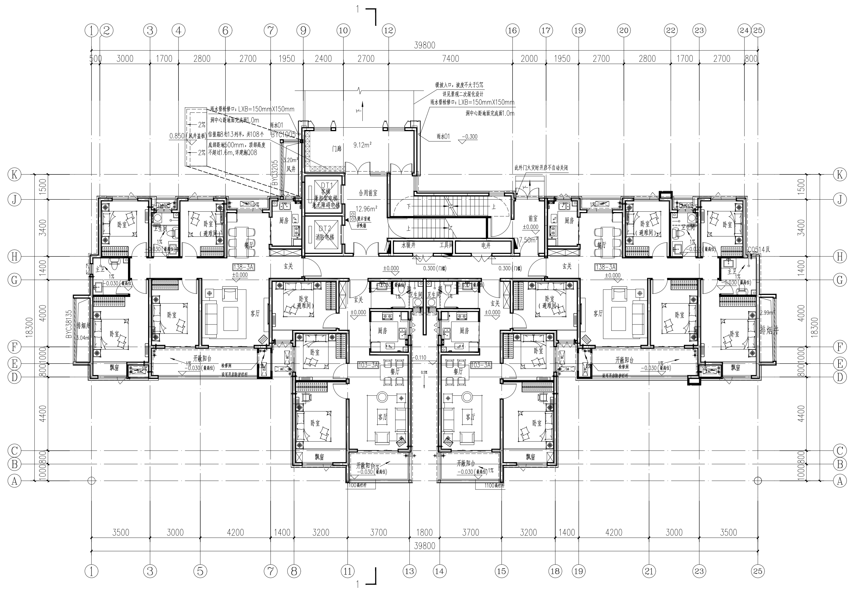
一层平面图 1:80
