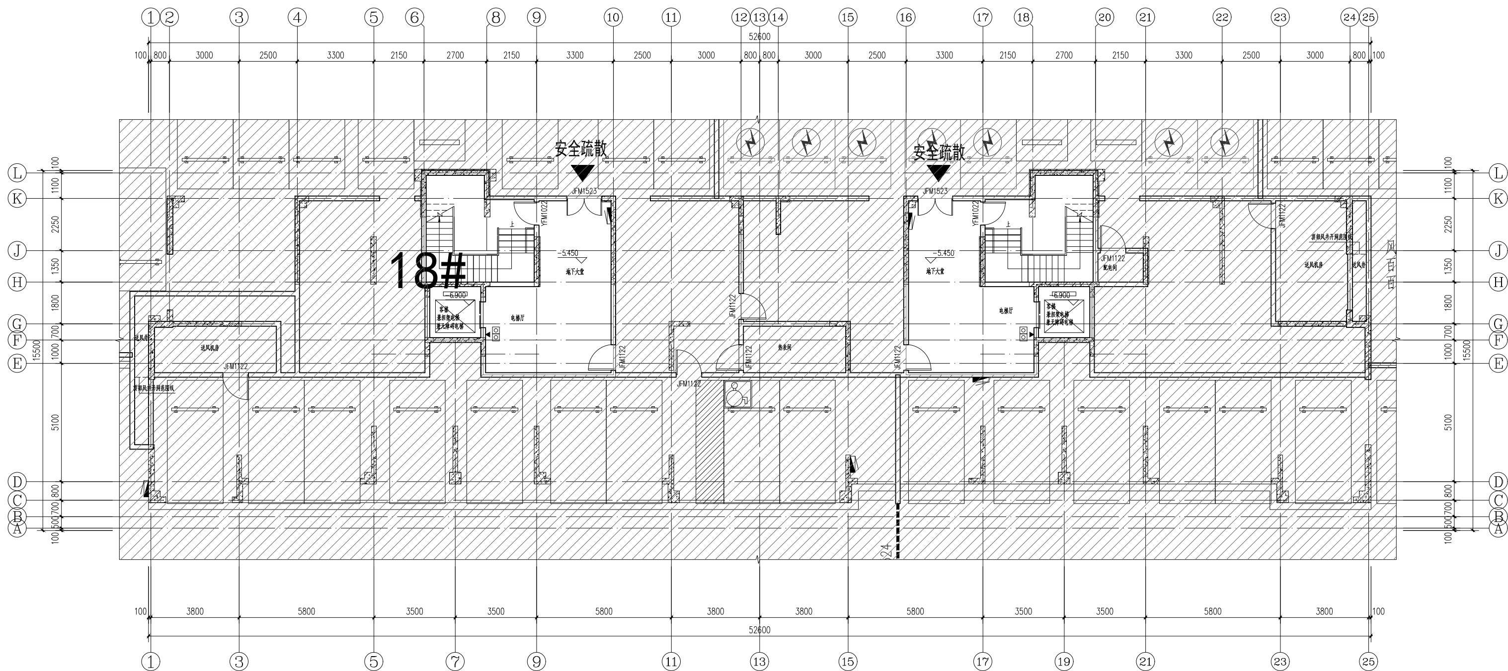
地下一层平面图 1:100
