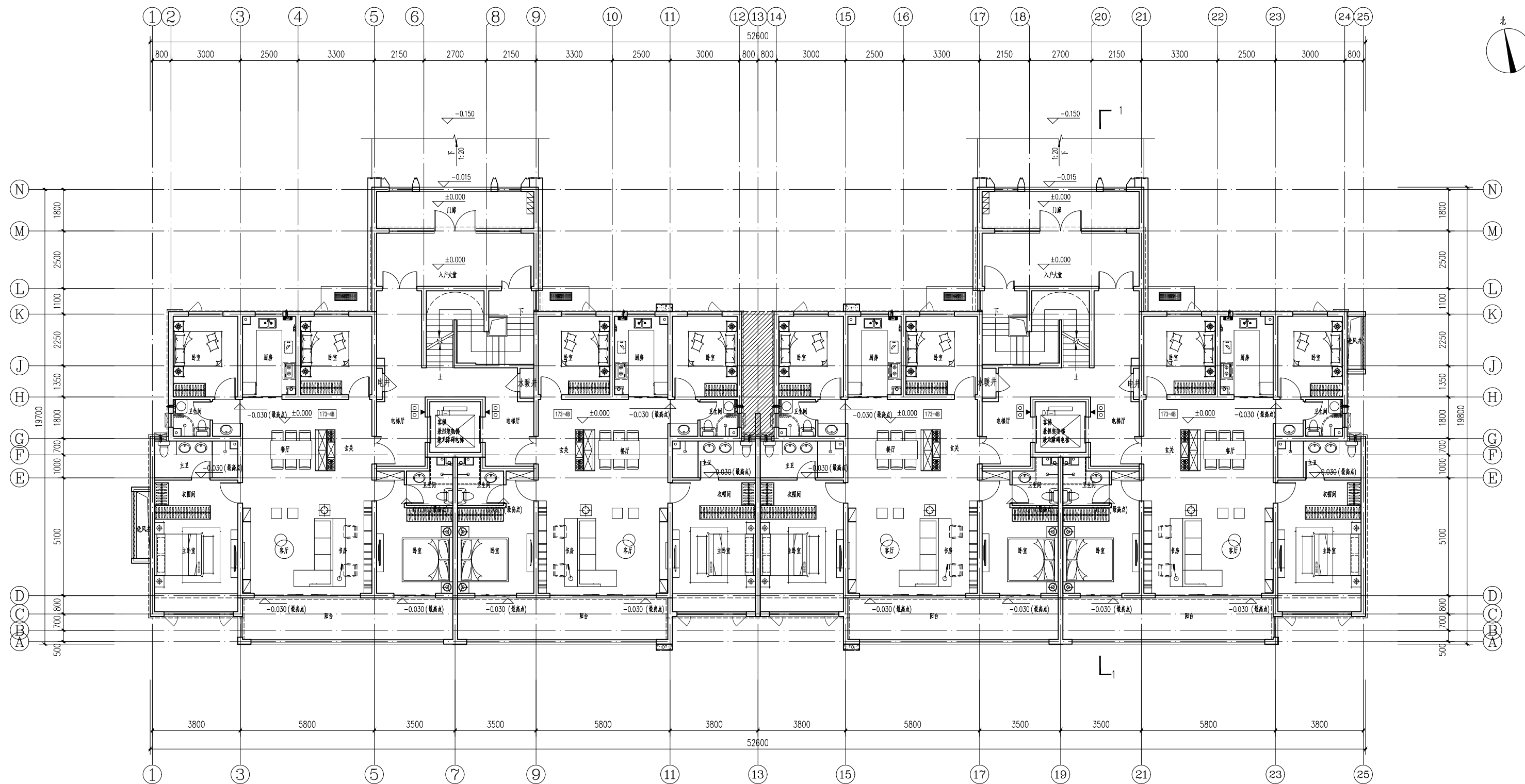
一层平面图 1:100
