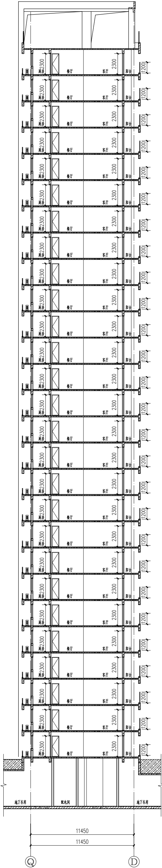
1-1 剖面图 1:150
