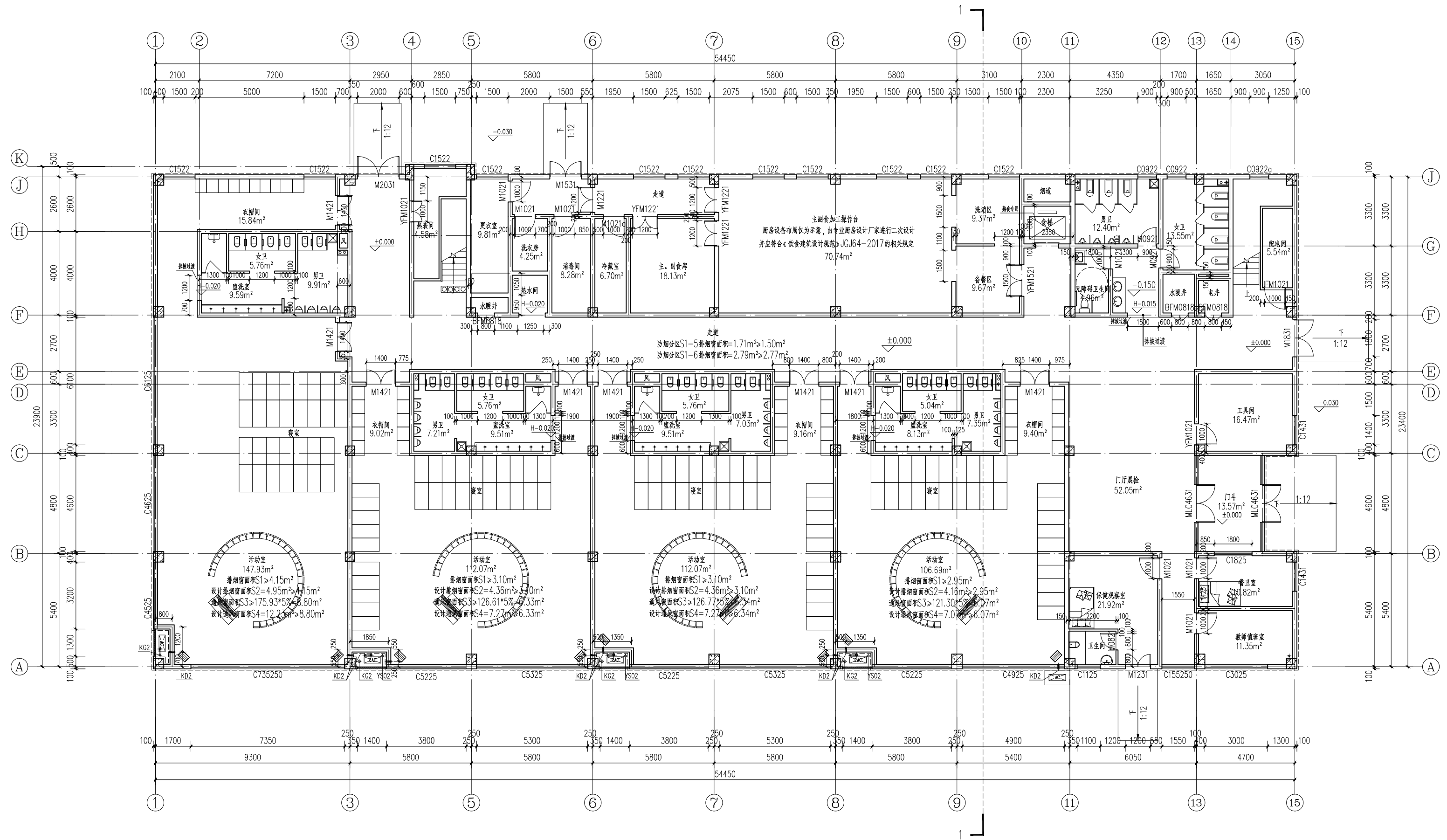
一层平面图 1:100
