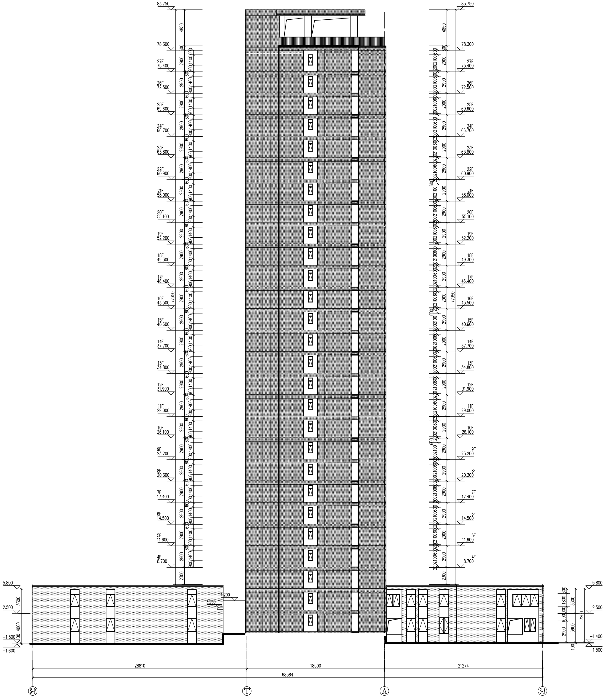
S-P ~ S-A 轴立面图 1:150
