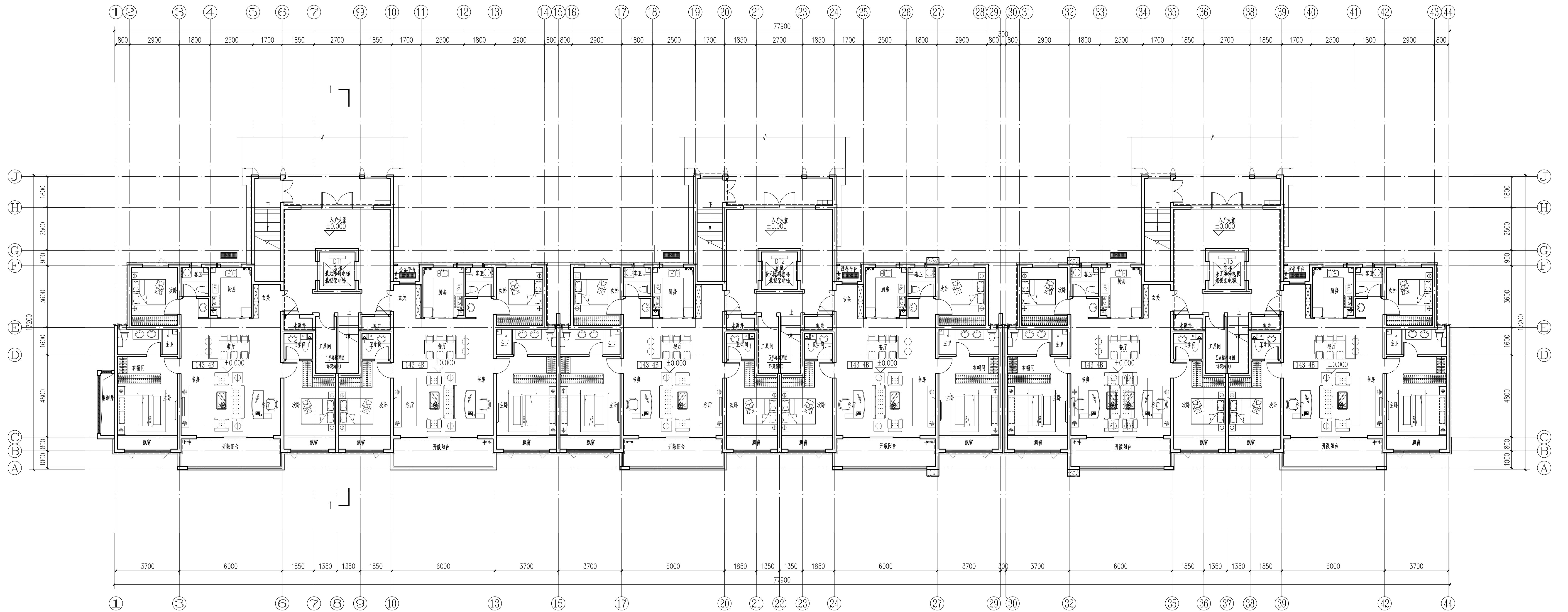
一层平面图 1:100 注：本层面积:935.54m 2
