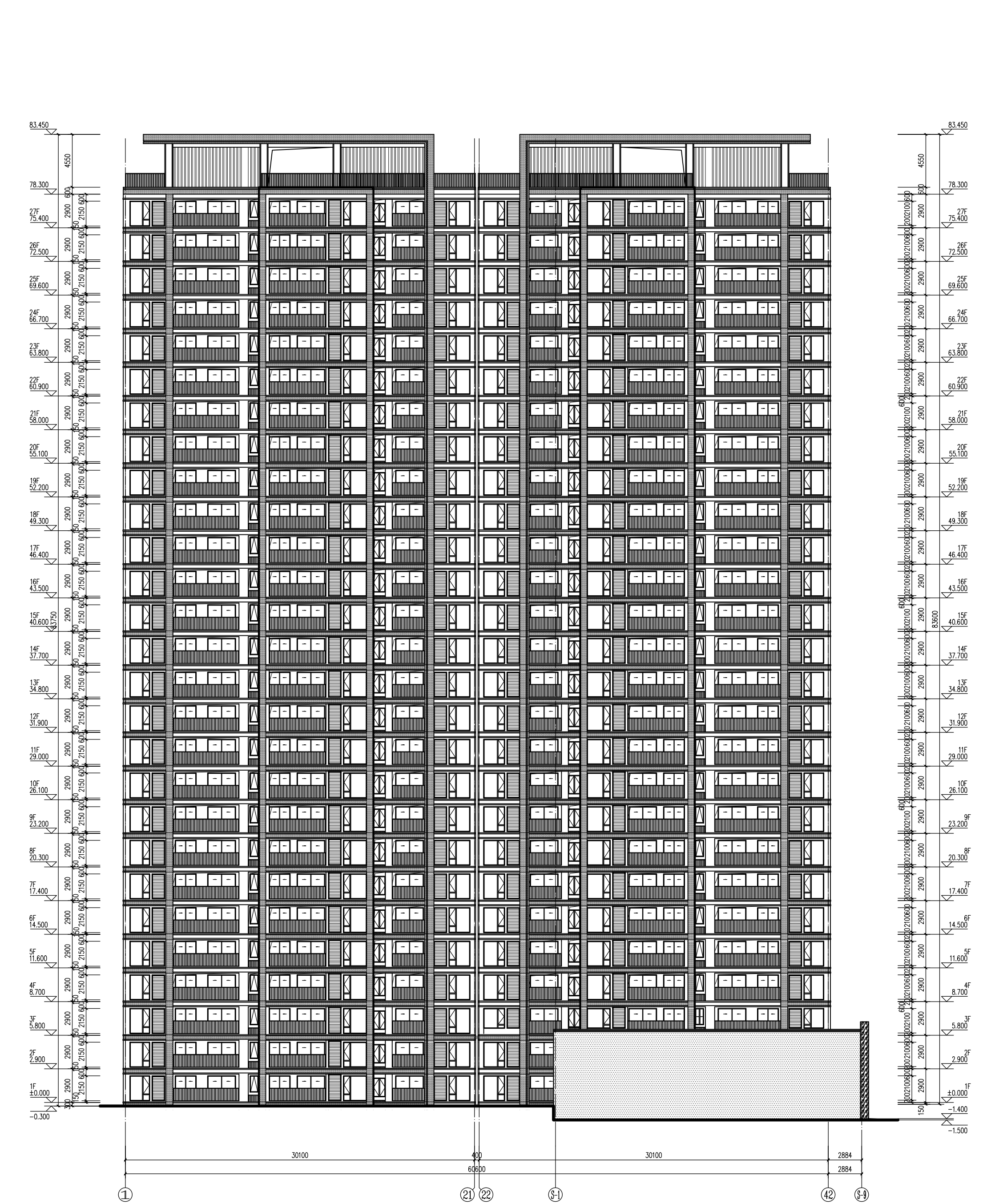
① ~ ④② 轴立面图 1:150
