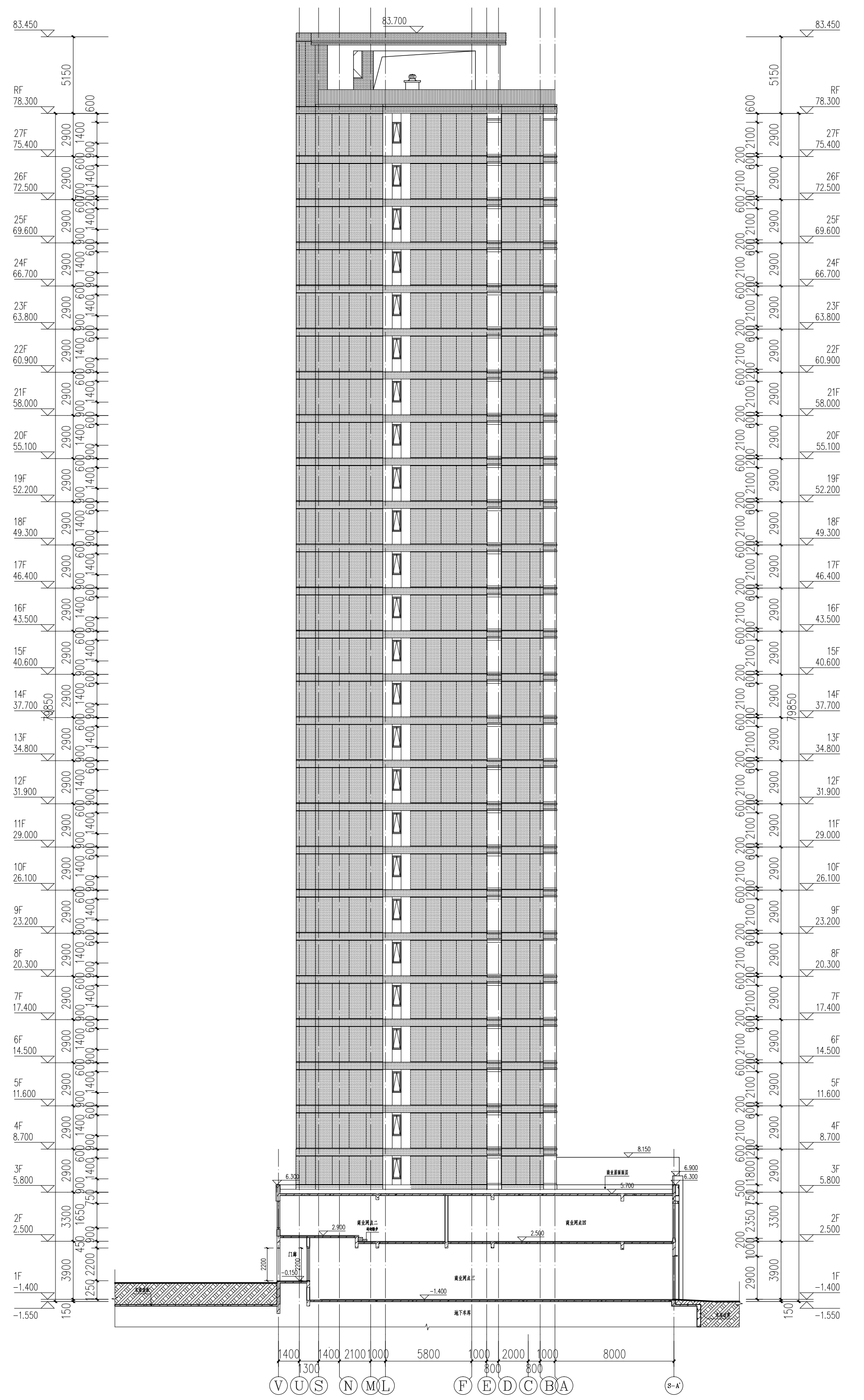
V~(5)立面图 1:200
