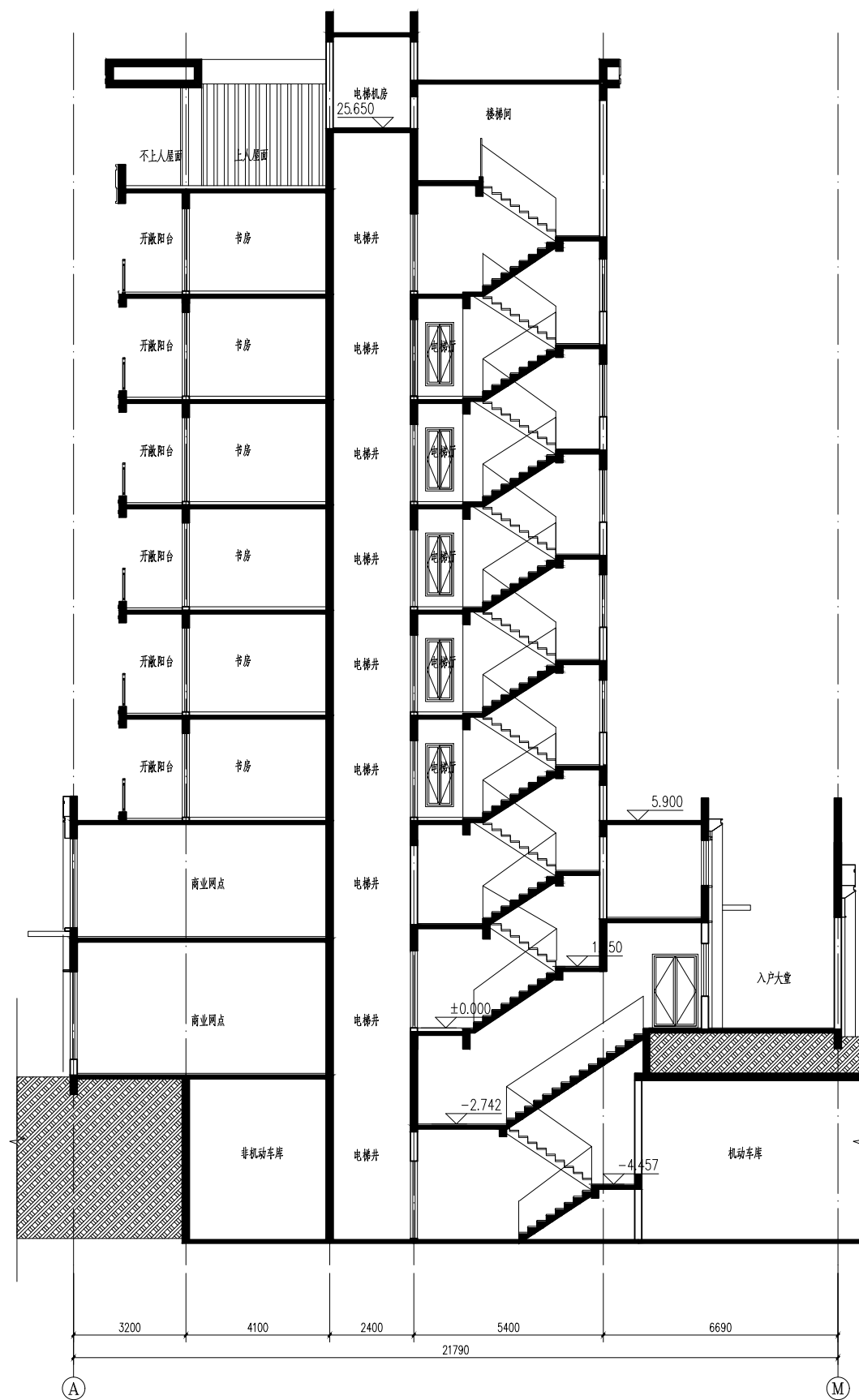
1-1剖面图 1:100
