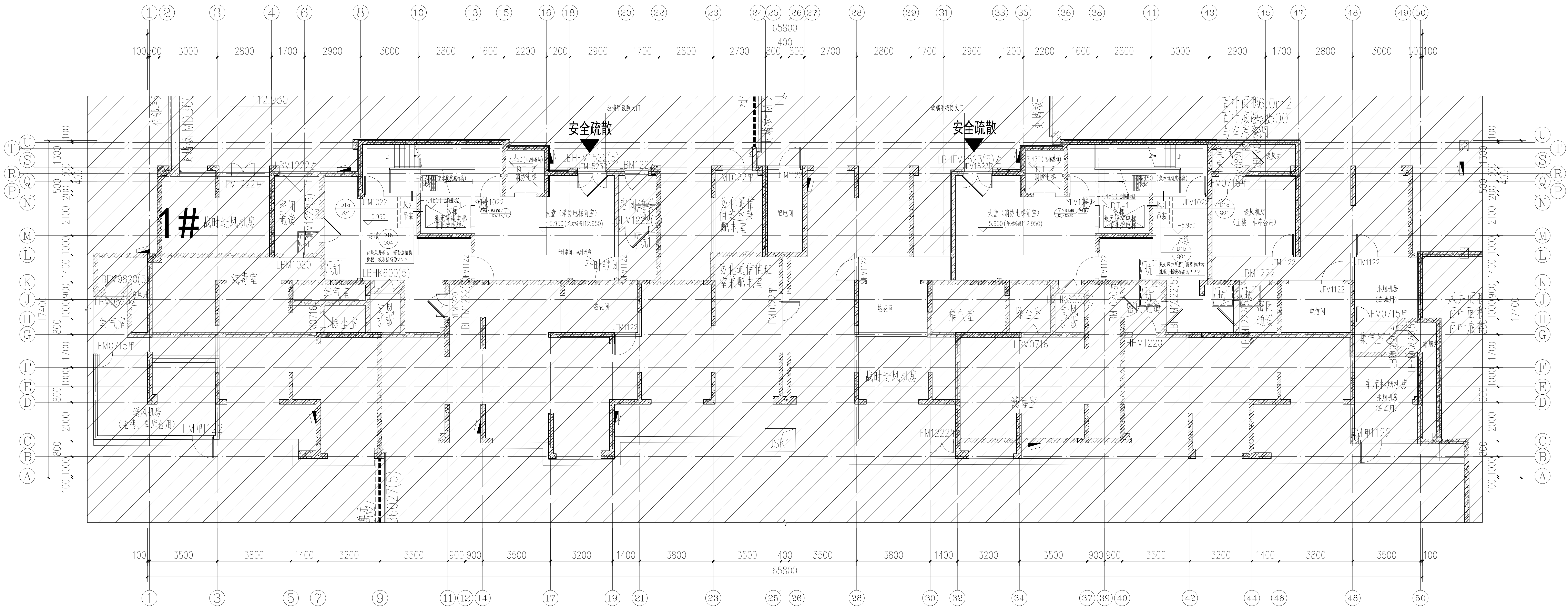
地下一层平面图 1:100
