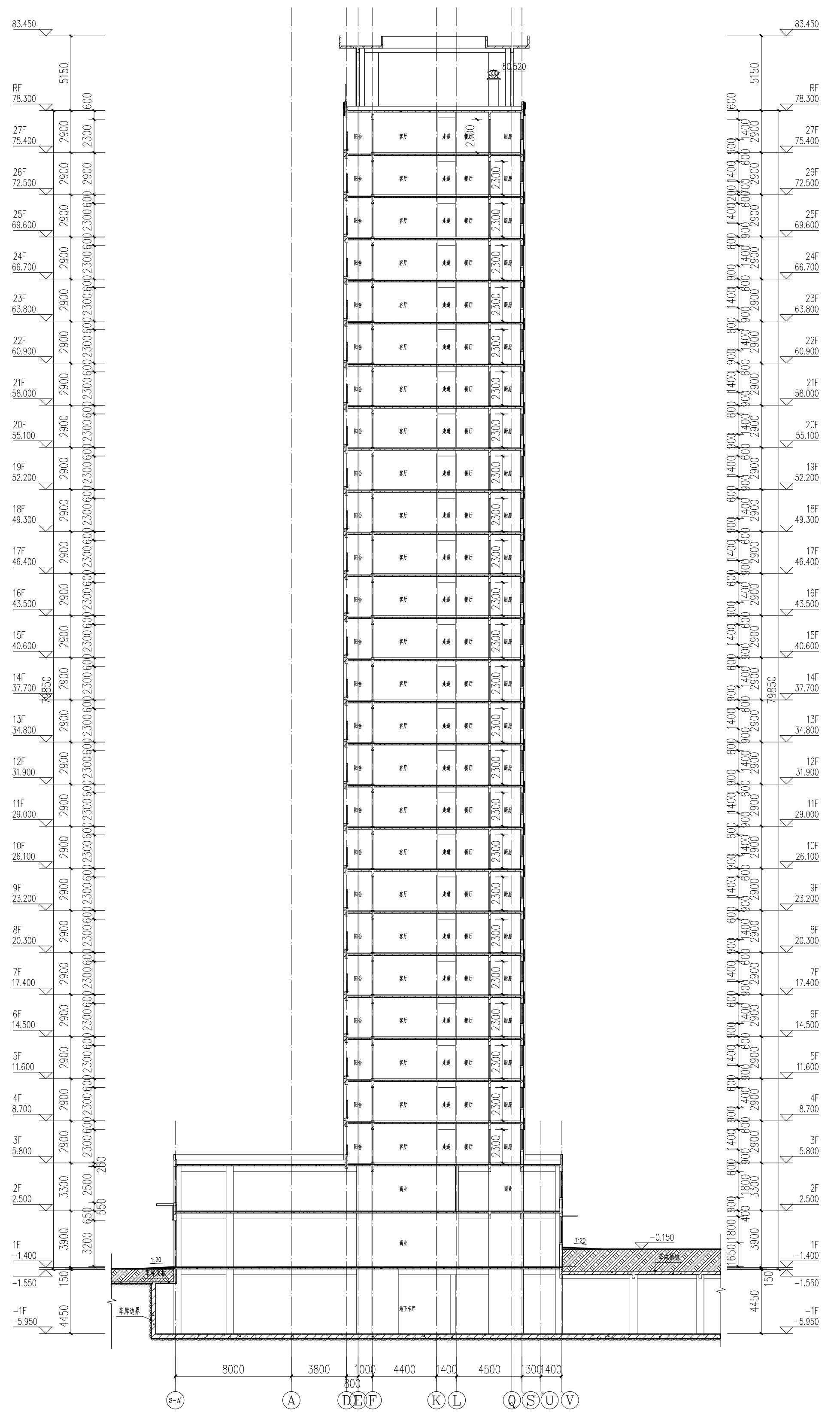
1-1剖面图 1:200
