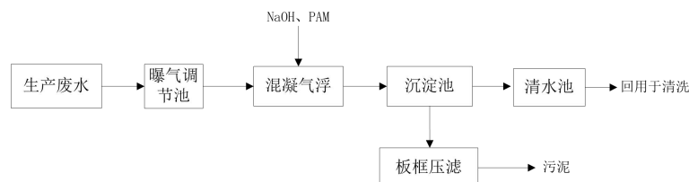
图 4-3 污水处理工艺流程图
