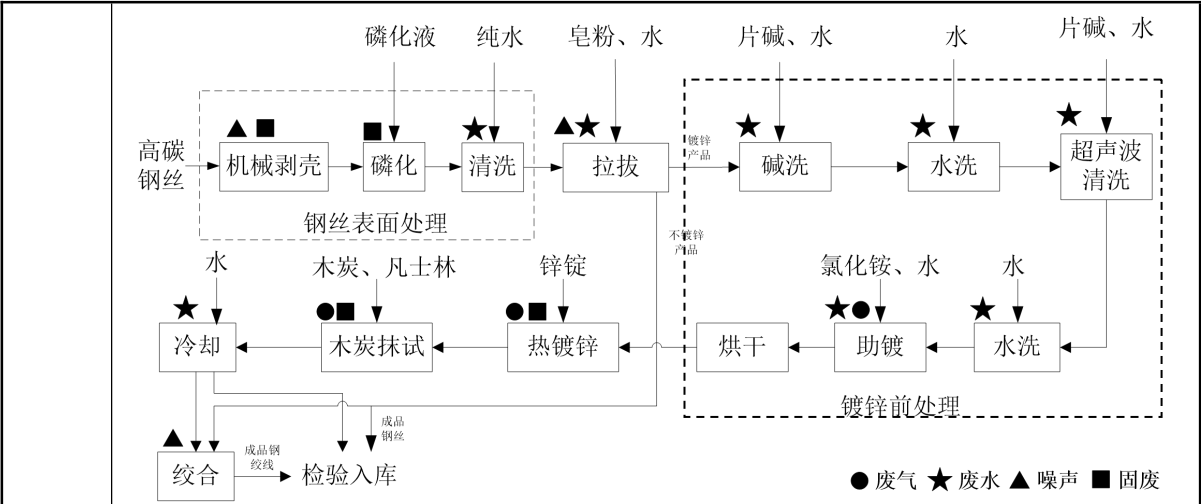
图 2-3 现有工程（一二车间生产线）工艺流程图
