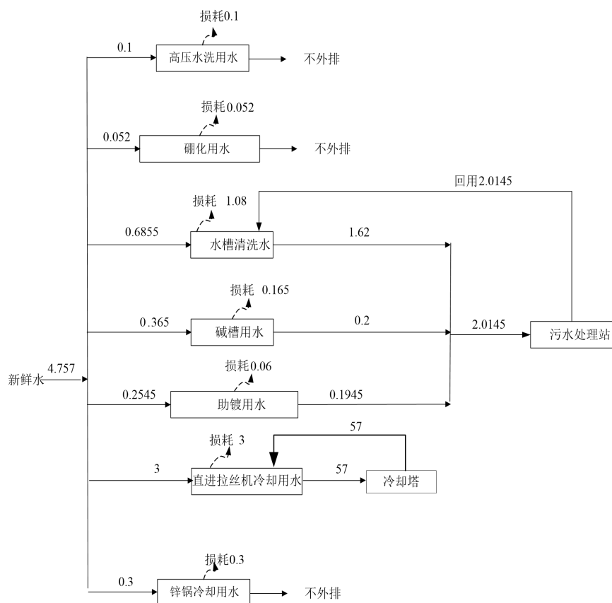
图 4-1 本项目用水量水平衡图 (m³/d)
